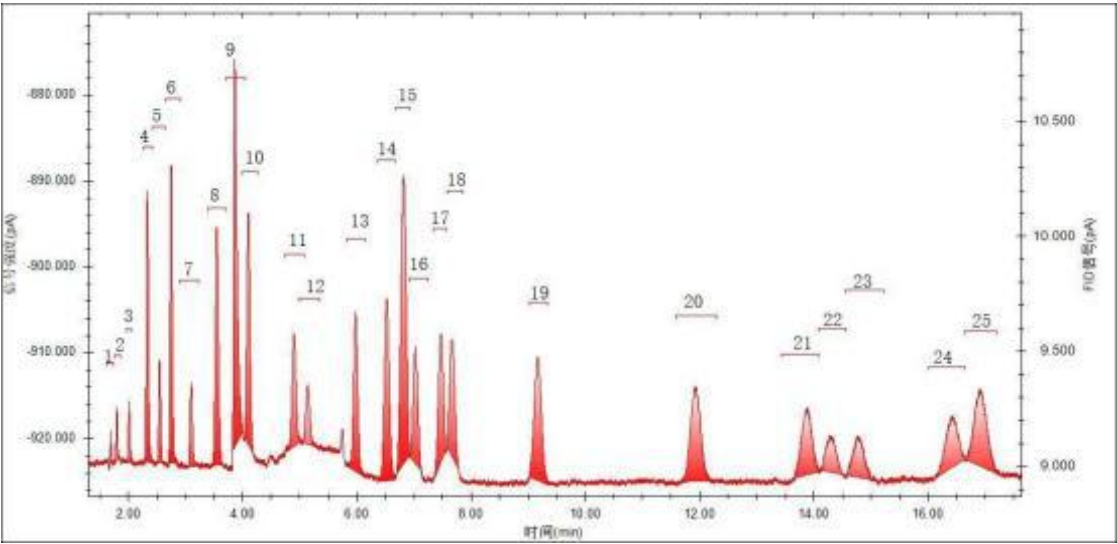
图1 便携式气相色谱仪测量20mg/m 3 的VOC物质谱图
